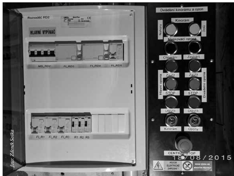
Hlavní jevištní rozvaděč a oponový ovládací pult
