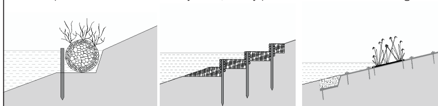
Obr. 2: Opevnění břehu: haťošterkový válec, vrbový plůtek a kokosová rohož s vegetací
