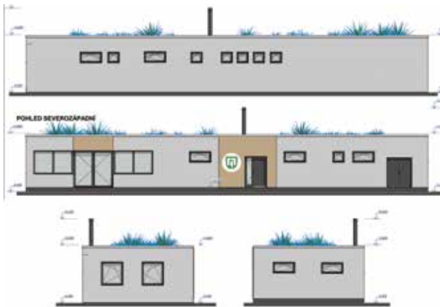
Aktuální verze budovy zázemí sportovního hřiště dle studie zpracované Ateliérem Ježek.
