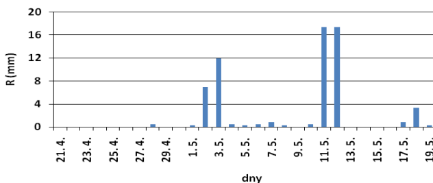
Průměrný denní úhrn srážek (mm) za období 21. 4. - 20. 5. 2013
