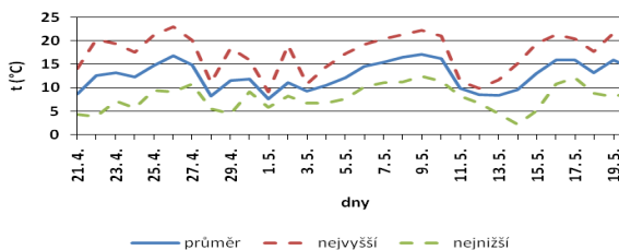
Chod průměrných teplot vzduchu (°C) v období 21. 4. - 20. 5. 2013
