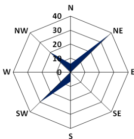
Průměrná četnost směrů větrů (%) za období 21. 4. - 20. 5. 2013
