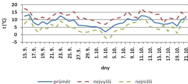
Chod průměrných teplot vzduchu (°C) v období 15. 9. - 21. 10. 2013
