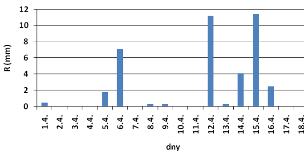
Průměrný denní úhrn srážek (mm) za období 1. 4. - 18. 4. 2012
