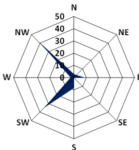
Průměrná četnost směrů větrů (%) za období 13. 9. - 17. 10. 2012
