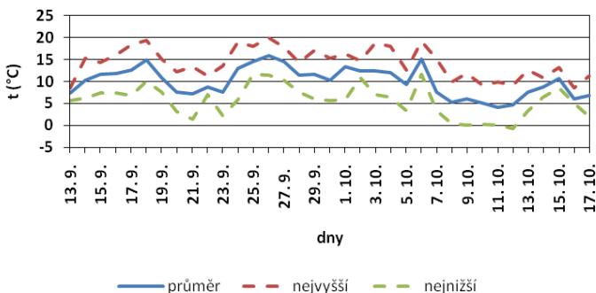
Chod průměrných teplot vzduchu (°C) v období 13. 9. - 17. 10. 2012
