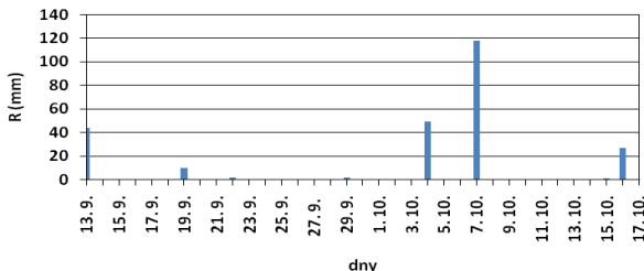
Průměrný denní úhrn srážek (mm) za období 13. 9. - 17. 10. 2012
